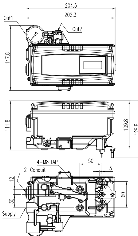
图2-13: YT-3303R (叉杆型)
