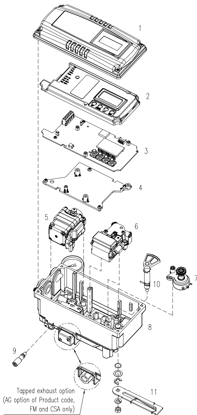
图2-2: YT-3303分解图
