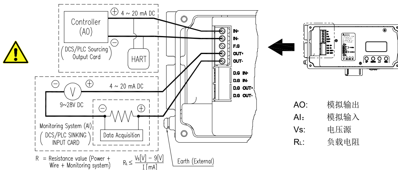
图5-1：标准端子概览
