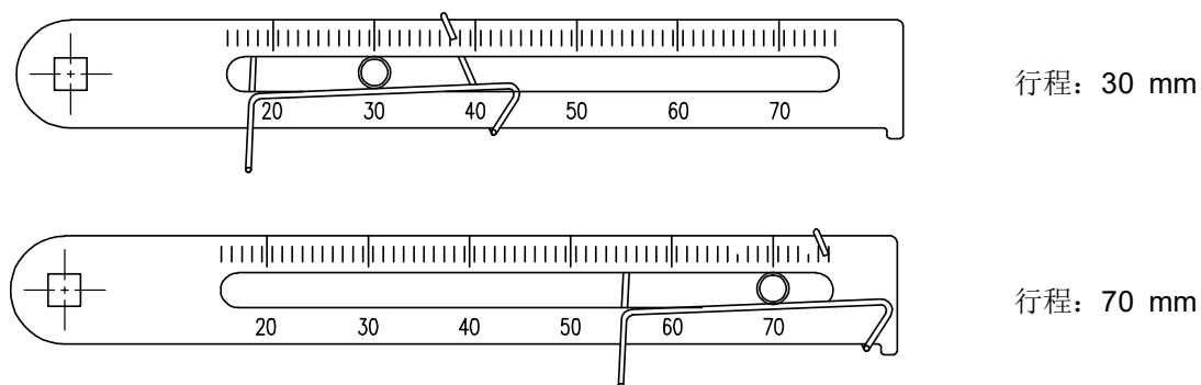
图3-14: YT-3303L / 3301L反馈杆和连接杆的位置
