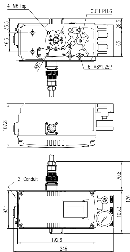
图2-17: YT-3301定位器
