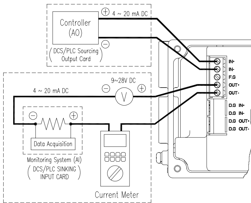
图9-3：设置发送器
