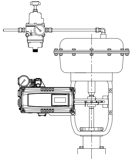
图3-9: YT-3303L / 3301L
