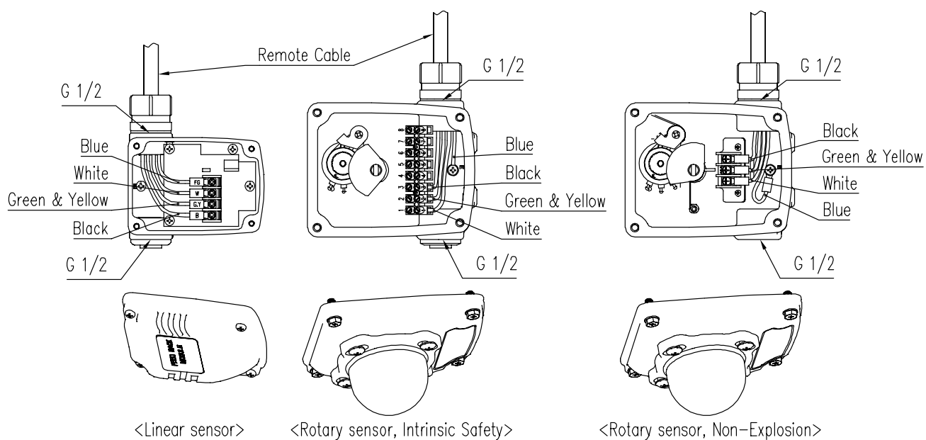
图5-4： 远程传感器和电缆（仅YT-3301L）
