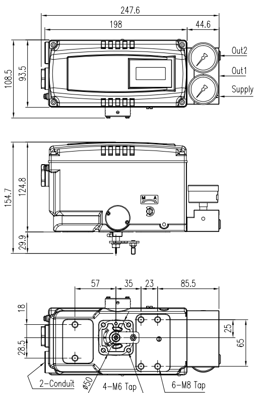
图2-10: YT-3350R (叉杆型)
