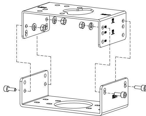
图3-28: 支架分解图
