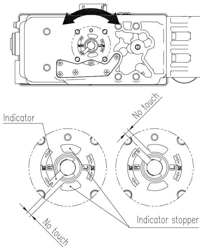
图3-33: 指标不得触及阀门行程0 % ~ 100 %处的指标止动件
