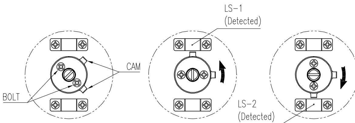
图6-2: 感应式 接近型
