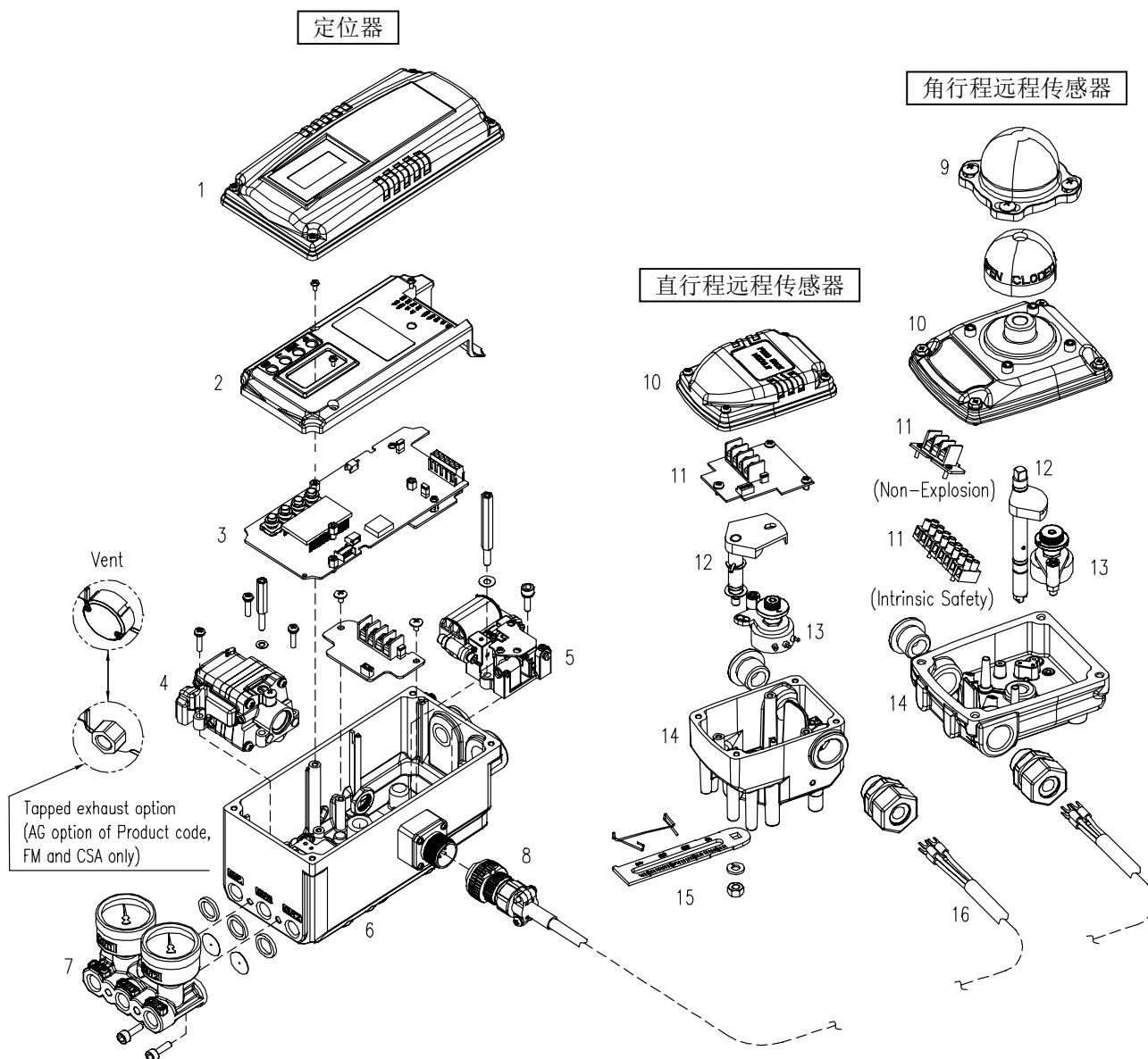
图2-3: YT-3301分解图
