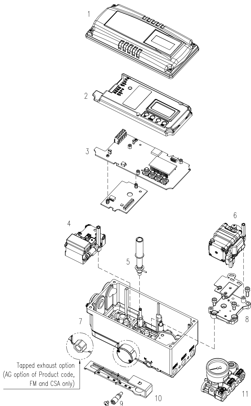
图2-1: YT-3300 / 3350分解图
