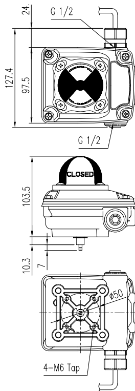
图2-16: 角行程远程传感器
